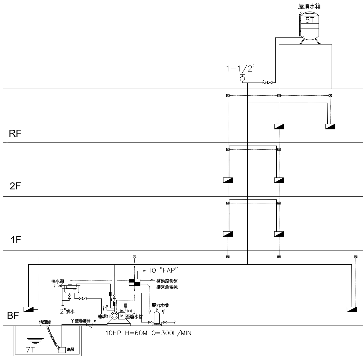
消防系統異位圖
